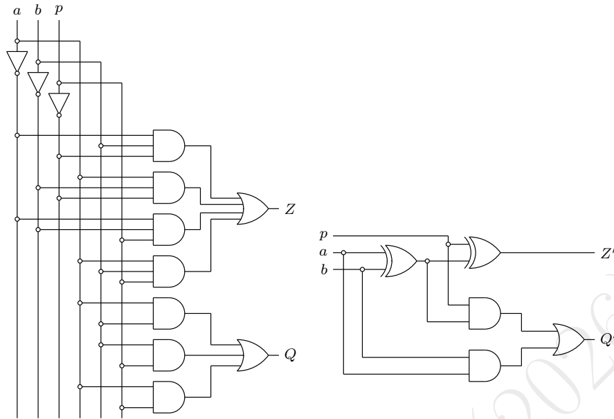
Slika 8.7: Osnovni i optimizovani dizajn sabirača.
