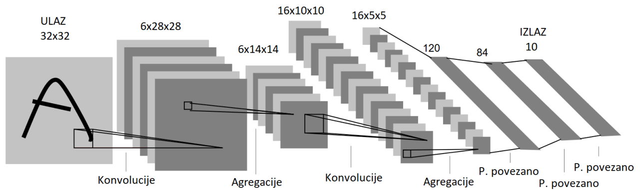
Slika 12.9: Arhitektura mreže LeNet-5.
