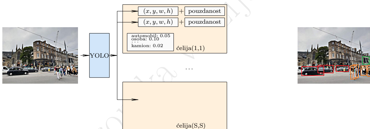
Slika 12.12: Shema modela pridruženog ćeliji.
