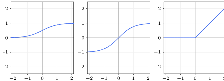
Slika 12.4: Sigmoidna funkcija, hiperbolički tangens i ispravljena linearna jedinica.
