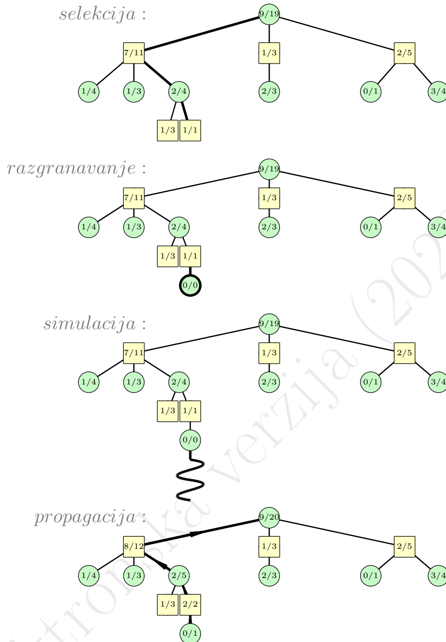
Slika 5.6: Ilustracija primene Monte Karlo pretrage stabla igre.
