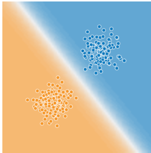
Slika 12.3: Podaci koji se sastoje od dve klase i prava koja ih razdvaja. Boje ukazuju na regione prostora koji pripadaju različitim klasama, a bela prava u centralnom delu odgovara uslovu P(y = 1|\mathbf{x}) = f_{\mathbf{w}}(\mathbf{x}) = 0.5 (slika je generisana pomoću alata A Neural Network Playground).
