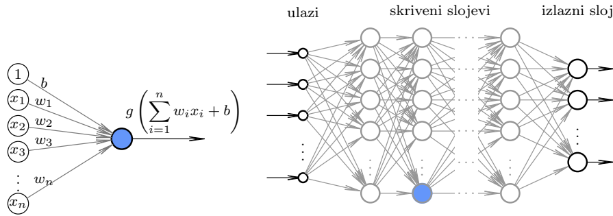
Slika 12.5: Struktura neurona i arhitektura potpuno povezane neuronske mreže.
