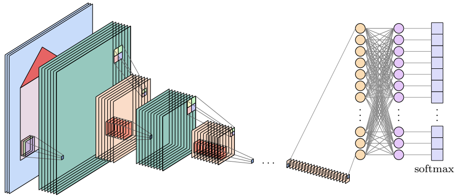
Slika 12.7: Shema konvolutivne neuronske mreže. Konvolutivni slojevi su prikazani zelenom bojom, a slojevi agregacije narandžastom. Na desnoj strani je prikazana potpuno povezana mreža bez skrivenih slojeva kojom se konvolutivna mreža završava. Prvi, narandžasti element predstavlja preoblikovanu formu poslednjeg izlaznog tenzora u obliku u kojem potpuno povezana mreža može da ga prihvati kao svoj ulaz. Drugi, ljubičasti element predstavlja rezultat linearne transformacije nad narandžastim delom, a poslednji element predstavlja rezultat primene funkcije softmax nad prethodnim.
