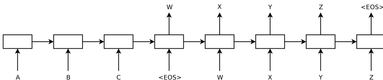
Slika 12.15: Ilustracija enkoder-dekoder arhitekture. Slova A , B i C predstavljaju ulazne reči, a W , X , Y i Z izlazne reči, a EOS kraj sekvence.
