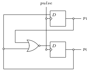
Slika 8.8: Dizajn brojača koji broji ciklično od 0 do 2.
