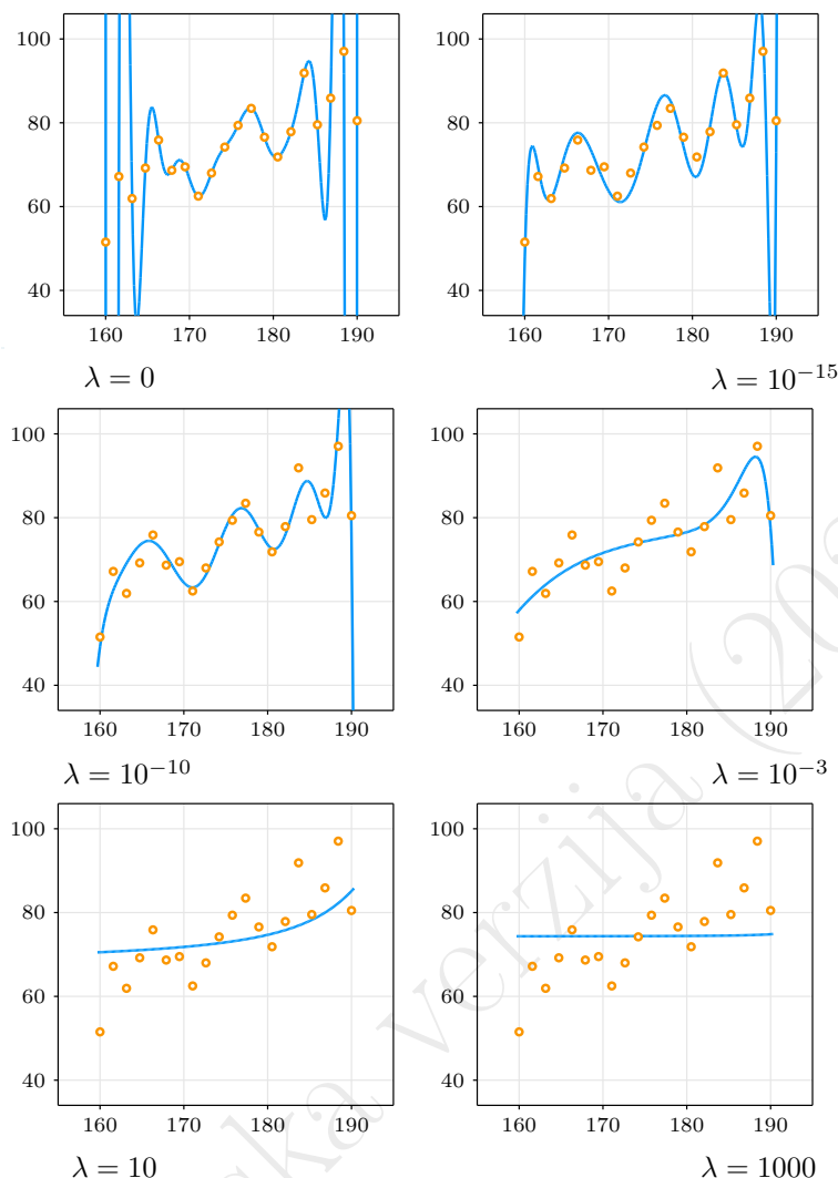
Slika 12.1: Polinomski modeli stepena 19 dobijeni za različite vrednosti regularizacionog hiperparametra.
