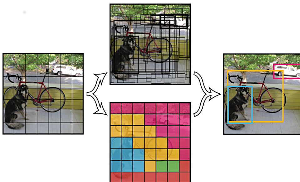
Slika 12.11: Ilustracija rada YOLO mreže. Levo je prikazana ulazna slika izdijeljena na ćelije. Dole su različitim bojama prikazane različite klase objekata koji se prepoznaju u svakoj ćeliji. Gore su prikazana predviđanja svih pravougaonika koji obuhvataju objekte, pritom se značajno preklapaju. Desno je prikazan finalni izlaz nakon izbora manjeg broja relevantnih pravougaonika.
