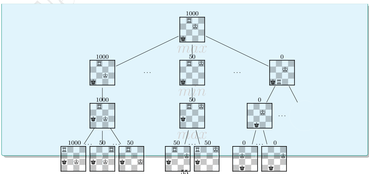
Slika 5.3: Algoritam Minimaks.
