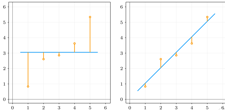
Slika 12.8: Grafici grešaka u odnosu na prosek (levo) i u odnosu na model (desno).
