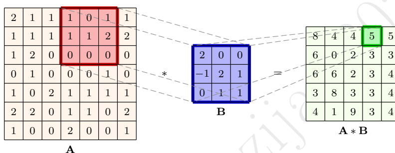
Slika 12.6: Ilustracija konvolucije: element rezultujuće matrice u zelenom polju dobija se kao skalarni proizvod crveno obojenog dela matrice \mathbf{A} i matrice \mathbf{B} . Ostatak rezultujuće matrice dobija se analogno. U opštem slučaju matrice ne moraju biti kvadratne.
